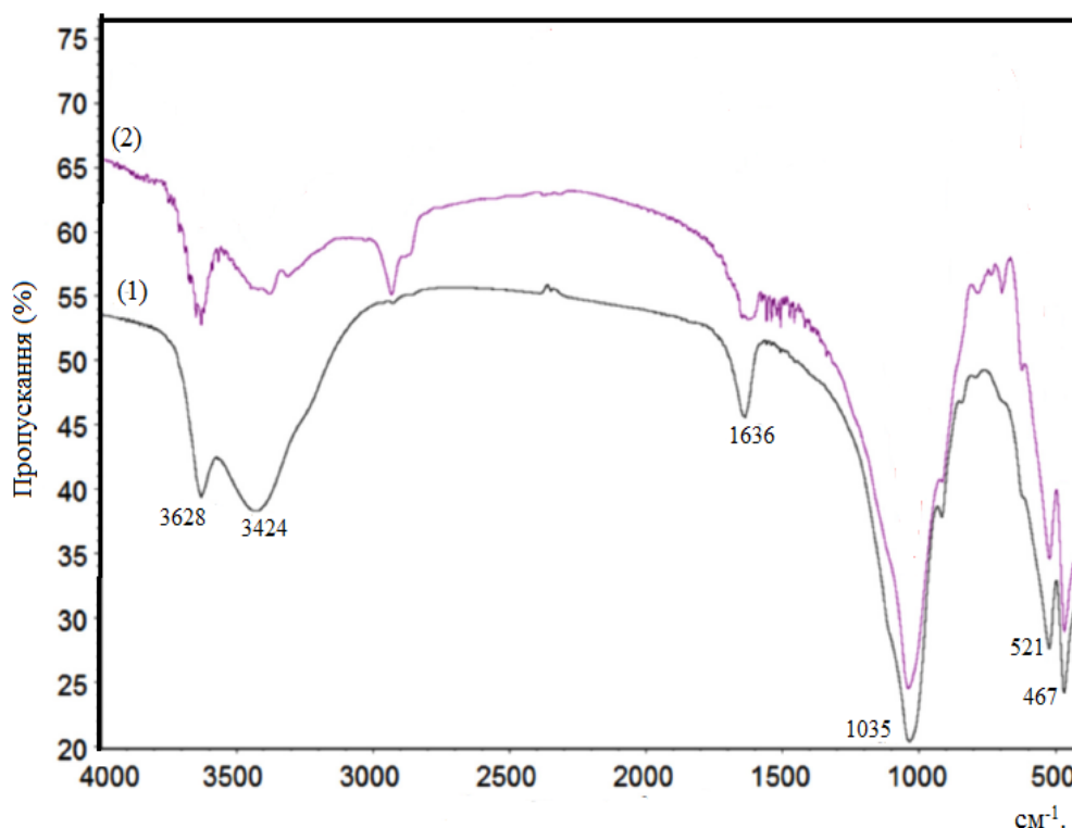
Рисунок 3.2 - ІЧ-спектри вихідного (1) та поверхнево-модифікованого монтморилоніту в толуолі (2)
