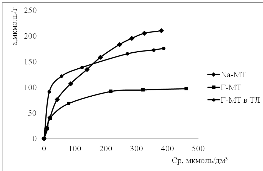
Рисунок 4.1 - Ізотерми сорбції \text{Co}^{2+} на вихідному та поверхнево-модифікованих зразках монтморилоніту (рН = 6)
