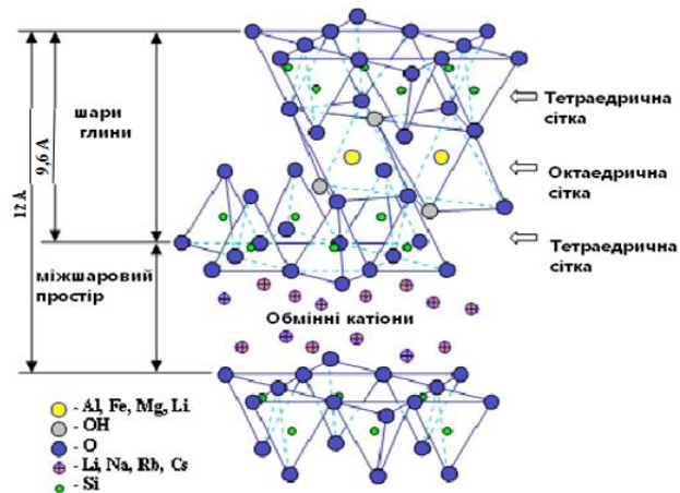
Рисунок 1.1 - Структура монтморилоніту
