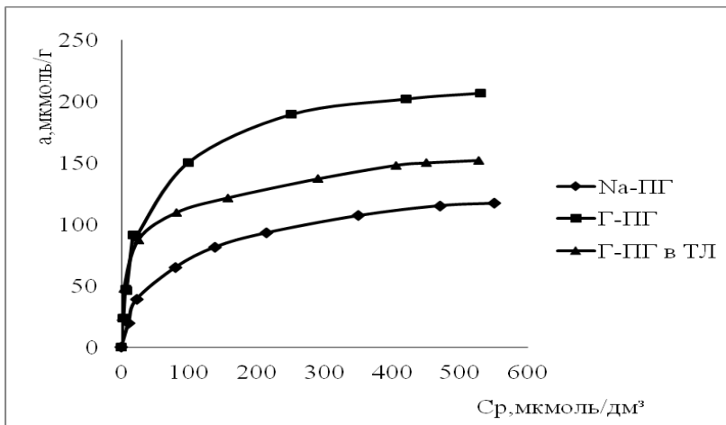
Рисунок 4.2 - Ізотерми сорбції Co^{2+} на вихідному та поверхнево-модифікованих зразках палигорськіту (рН=6)
